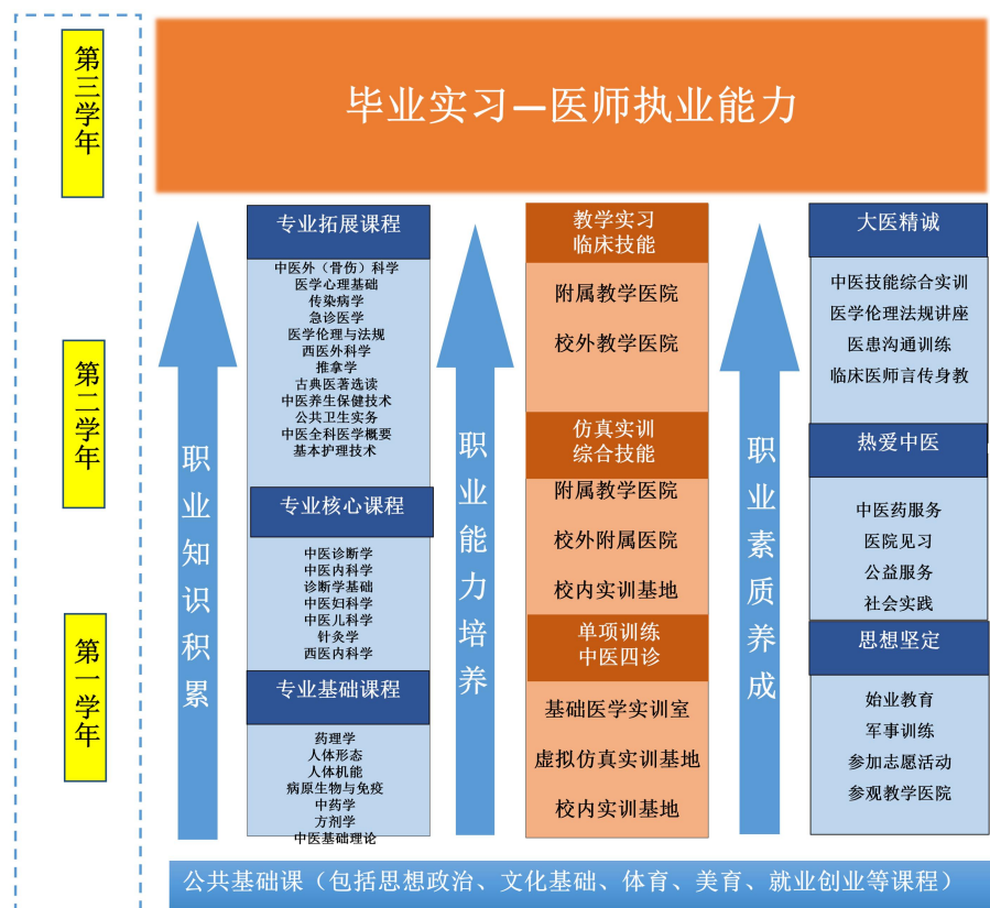
图 1 课程体系图
