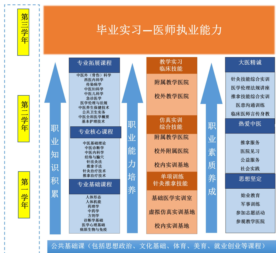
图1 课程体系
