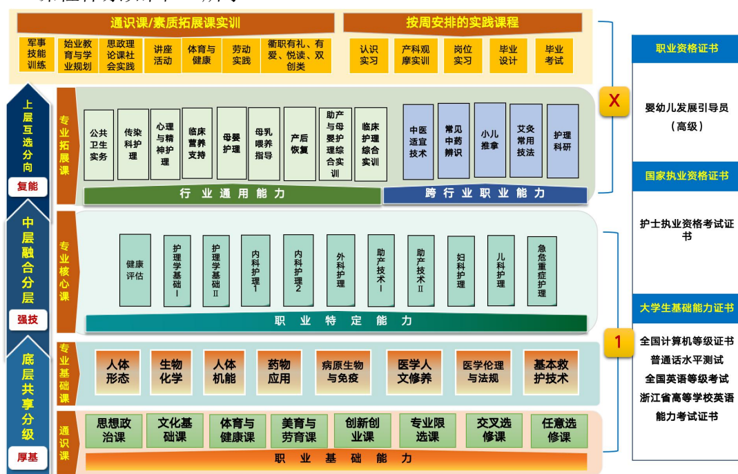
图1 课程体系图
