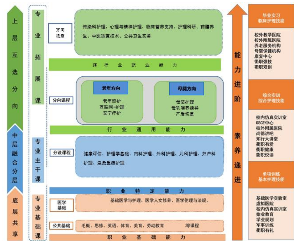
图 1 课程体系图
