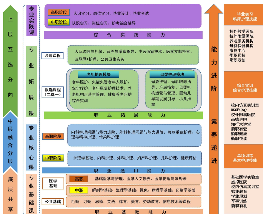
图 1 课程体系图
