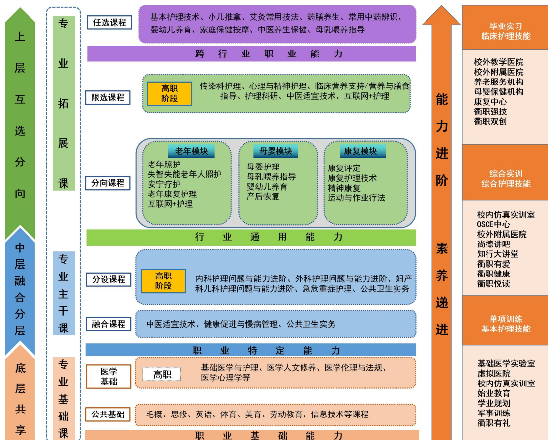
图 1 课程体系图
