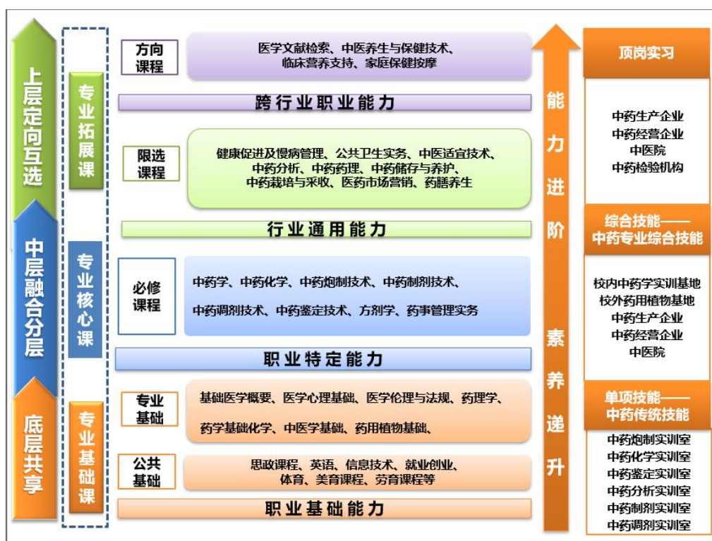
图 1 课程体系图
